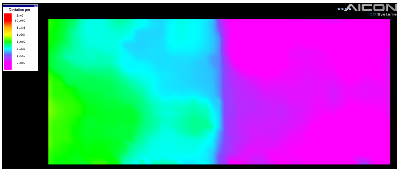
Abb. 1: Freundlich zur Verfügung gestellt von Herrn Hermstein, AICON 3D Systems GmbH Schichtstärken-Messung eines mit ReflexEx behandelten, gescannten Objekts
